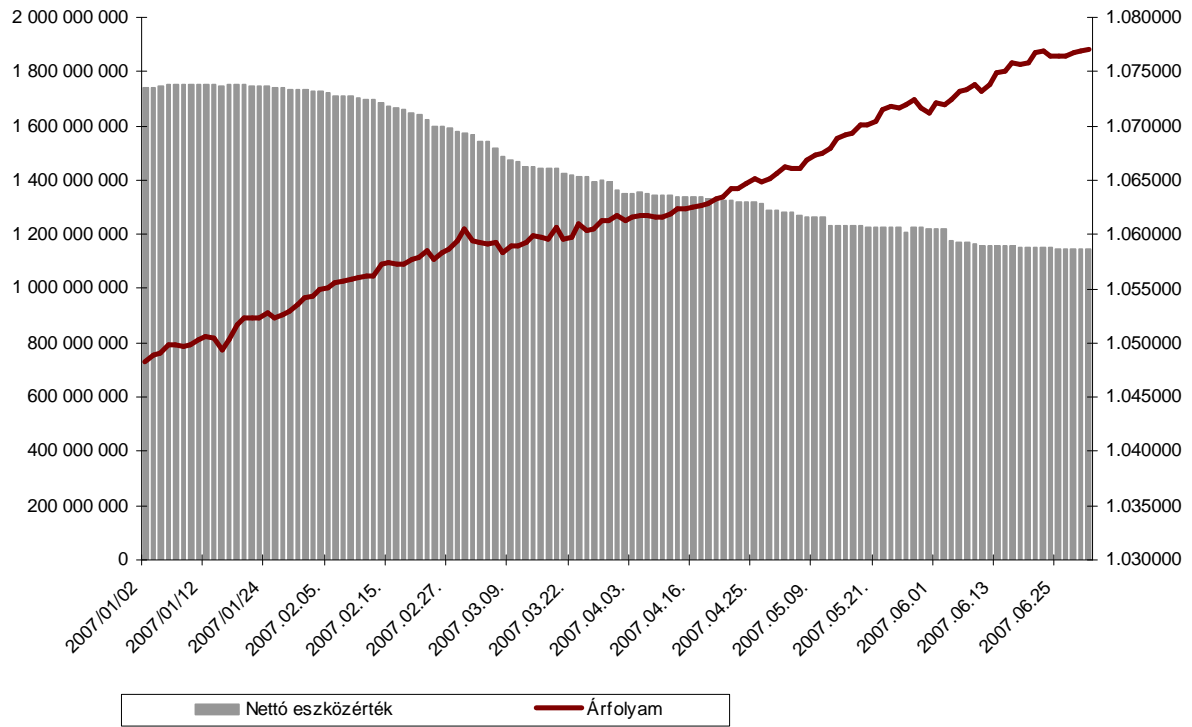
MKB Alapok Alapjanettó eszközértékének és egy befektetési jegyre jutó nettó eszközértékének alakulása 2007-01-02 és 2007-06-29 között. (1. sz. melléklet)
